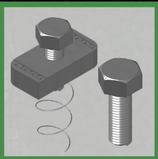
TUERCA RESORTE 3/8" PERNO 3/8"
