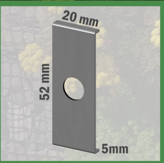
CORCHETE GALVANIZADO CON PERFORACIÓN
